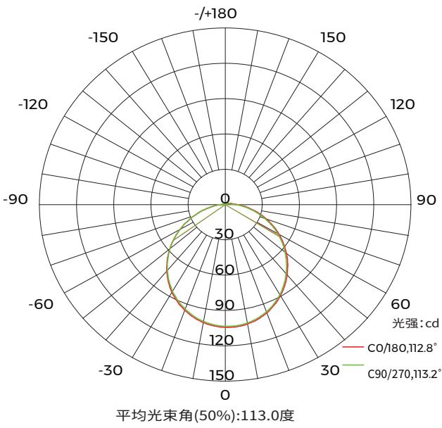
配光曲线
